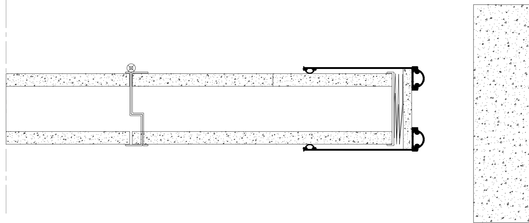
BİRLEŞİM DETAYI
