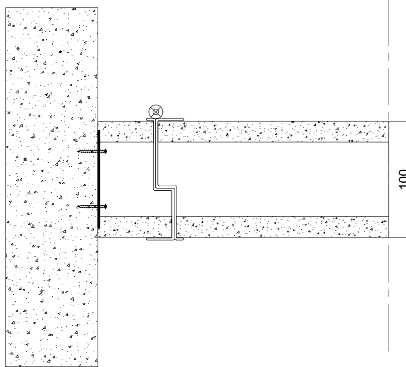
BAŞLANGIÇ DETAYI
